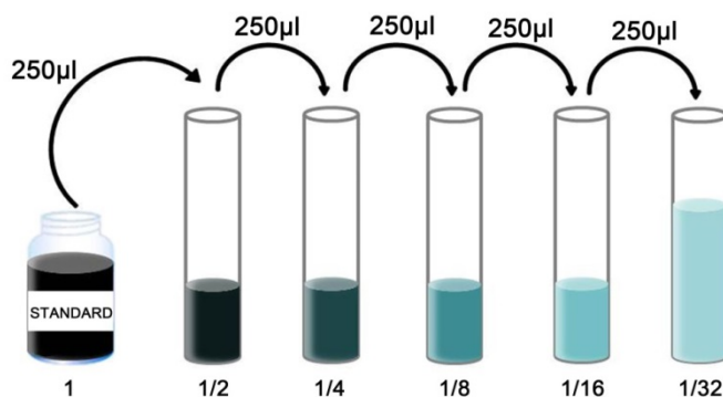
图2. 标准品倍比稀释示意图。按标准品(STANDARD)标签上标注体积加入标准品稀释液溶解并混匀后的浓度为标准品的起
